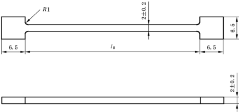
图 2 标准试样
