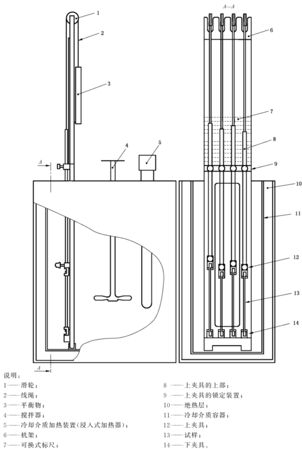
图1 回缩装置
